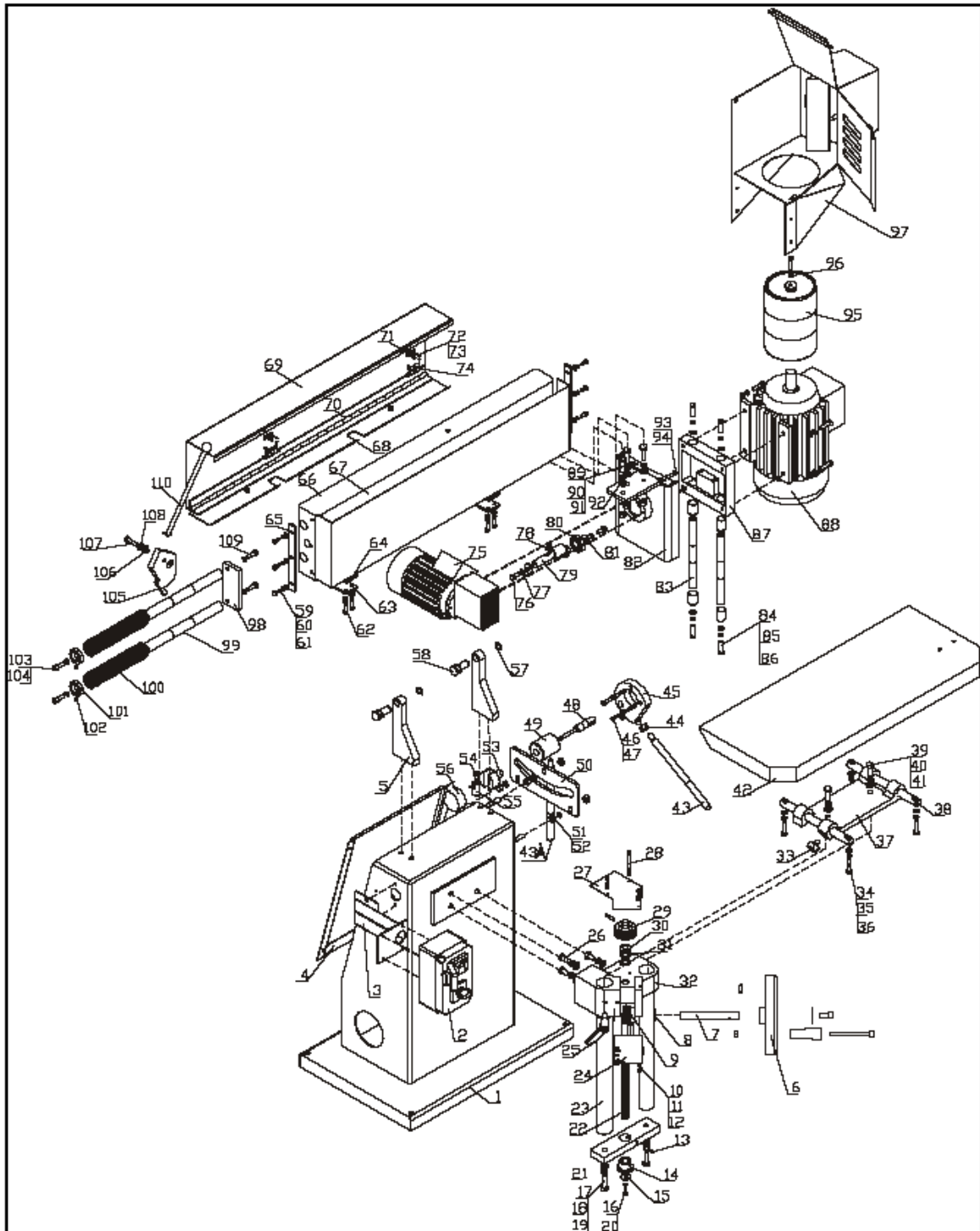
KSM2600.00.00.00 KANTENSCHLEIFMASCHINE
