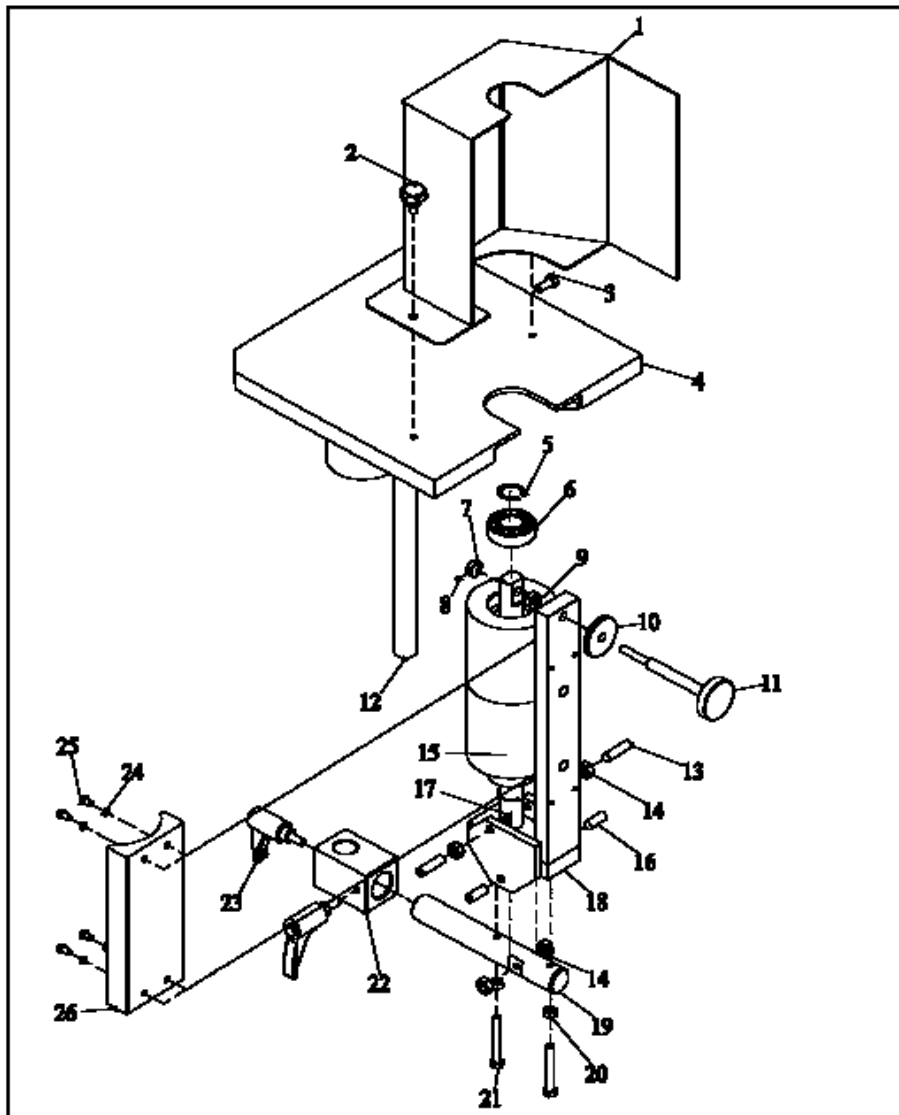
KSM3000.05.00.00 BEWIGLICHSATTEL
